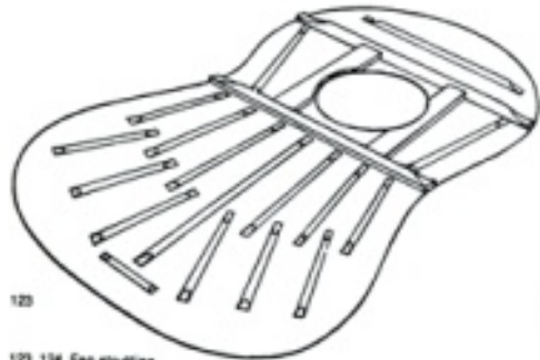
123, 124. Fan strutting.
